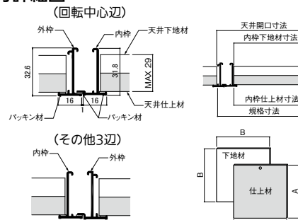
部分詳細図
