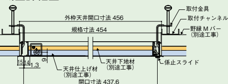
断面詳細図
